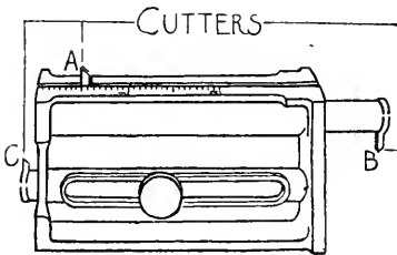
FIG. 35. BUTT GAGE.
